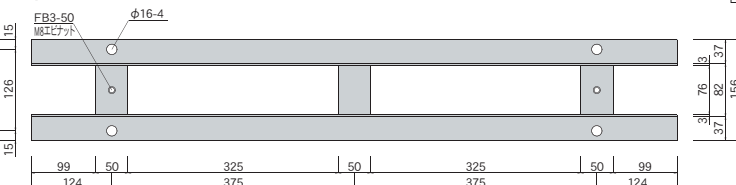
■平面図
