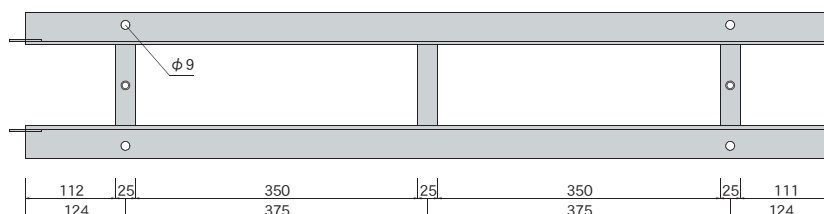
■固定式グレーチング：W95-H37
