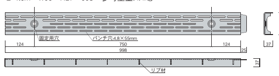
■固定式グレーチング：W95-H37
