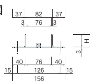
■断面図
