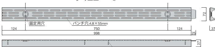
■固定式グレーチング：W72-H37（ペロ付き）
